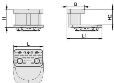
Конструктивные данные VCBL-B 120x50x48 TV
