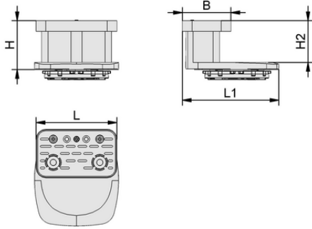
Tasarım verileri VCBL-B 125x75x48 TV
