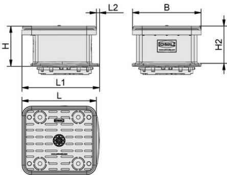
Datos de diseño VCBL-B 140x130x48 TV
