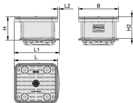
Données de construction VCBL-B 140x130x29 TV
