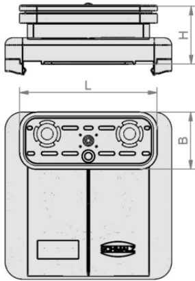
Tasarım verileri VCBL-S1 120x120x50 TV
