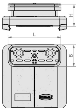
デザインデータ VCBL-S1 120x120x50 TV
