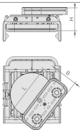
Dati di costruzione VCBL-K1 130x30x125 D-360
