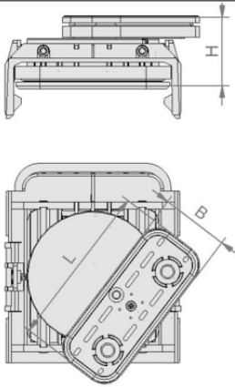
Tasarım verileri VCBL-K1 130x30x125 D-360
