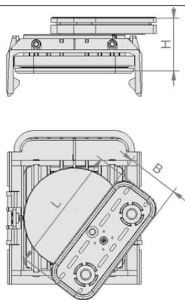
Données de construction VCBL-K1 130x30x125 D-360
