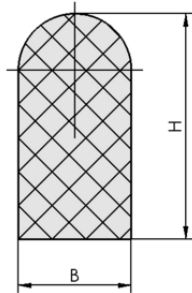
Tasarım verileri DR 188/180x6 MOS NK-20
