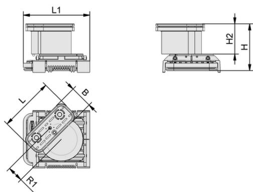
Données de construction VCBL-K2 120x50x125 D-360
