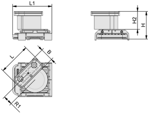
Tasarım verileri VCBL-K2 125x75x125 D-360
