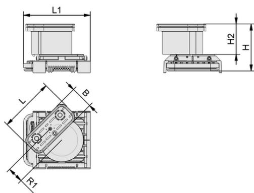
Dati di costruzione VCBL-K2 125x75x125 D-360
