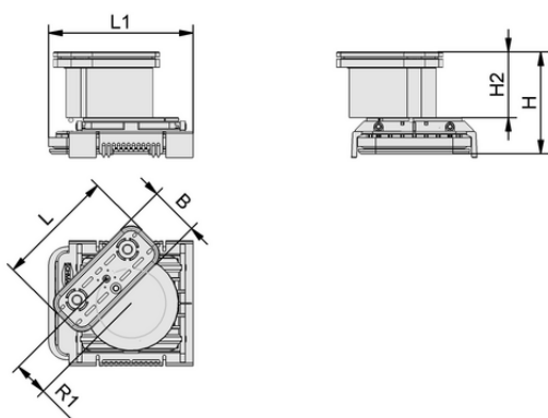
Données de construction VCBL-K2 125x75x125 D-360
