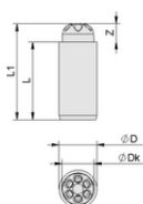
Конструктивные данные TV D9 4.3
