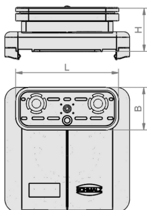
Dati di costruzione VCBL-S1 120x50x32.7 TV-S
