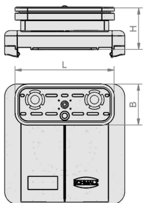
デザインデータ VCBL-S1 125x75x32.7 TV-S
