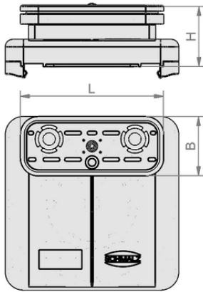
Tasarım verileri VCBL-S1 125x75x32.7 TV-S
