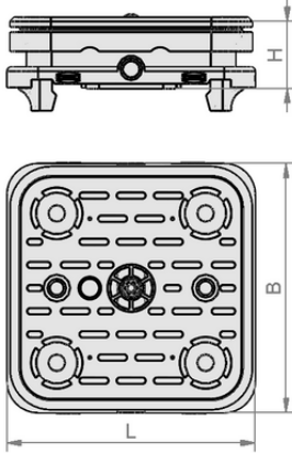
Tasarım verileri VCBL-S1 120x120x32.7 TV-S
