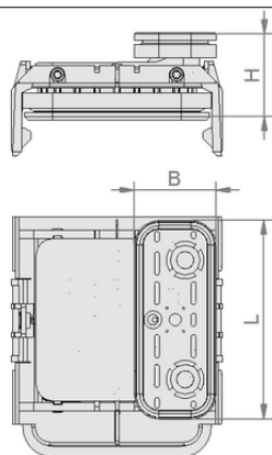
Конструктивные данные VCBL-K1 120x50x125 L
