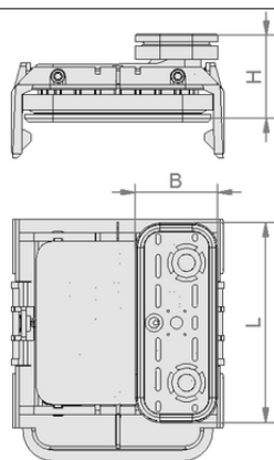
デザインデータ VCBL-K1 125x75x125 L
