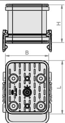
デザインデータ VCBL-K1 140x115x125
