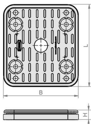
Dati di costruzione VCSP-O 140x130x16.5 TPE
