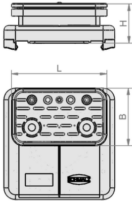
Tasarım verileri VCBL-S4 120x50x50 TV
