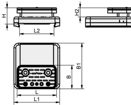
Tasarım verileri VCBL-S4 125x75x50 TV
