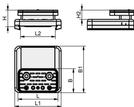
デザインデータ VCBL-S4 125x75x50 TV
