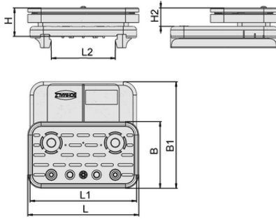
Tasarım verileri VCBL-S1 125x75x32.7 TV
