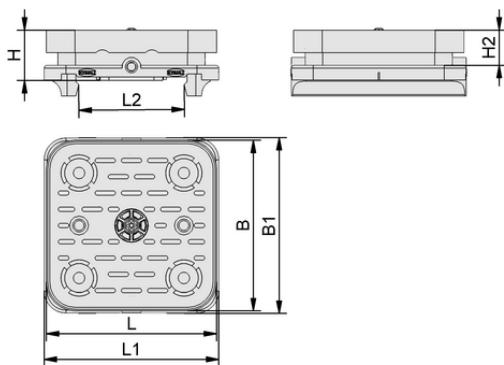
Konstruktionsdaten VCBL-S1 120x120x32.7 TV
