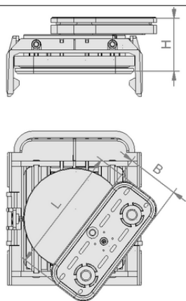
Dati di costruzione VCBL-K1 120x50x125 D-360
