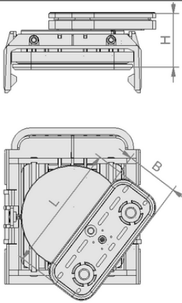
Tasarım verileri VCBL-K1 120x50x125 D-360
