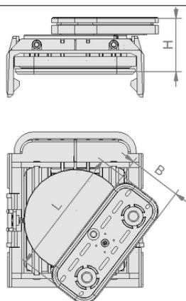
Dati di costruzione VCBL-K1 125x75x125 D-360
