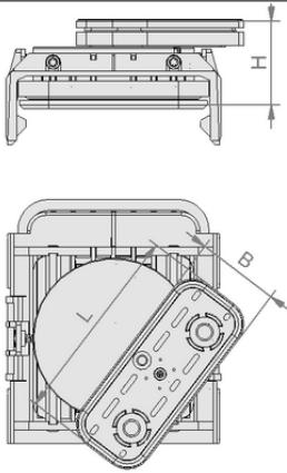
Tasarım verileri VCBL-K1 125x75x125 D-360
