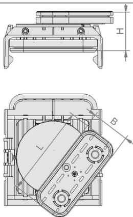
Datos de diseño VCBL-K1 125x75x125 D-360
