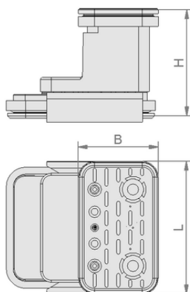
Dati di costruzione VCBL-K2 125x75x75 Q
