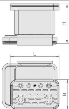
Données de construction VCBL-K2 120x50x125 L
