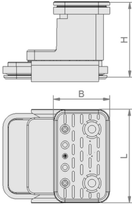
Tasarım verileri VCBL-K2 125x75x125 Q
