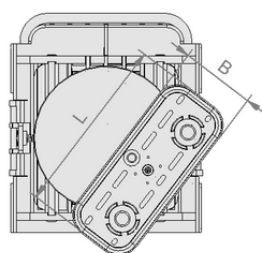
Конструктивные данные VCBL-K1 125x75x85 D-360
