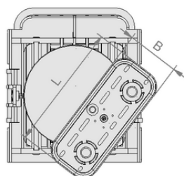
Données de construction VCBL-K1 125x75x85 D-360
