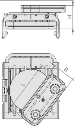
Tasarım verileri VCBL-K1 125x75x85 D-360
