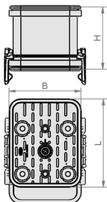
Données de construction VCBL-K1 140x115x85
