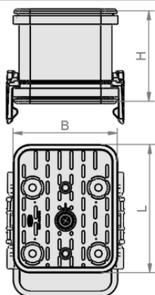
Конструктивные данные VCBL-K1 140x115x85
