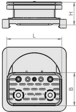
Tasarım verileri VCBL-S4 130x30x50 D-360 TV
