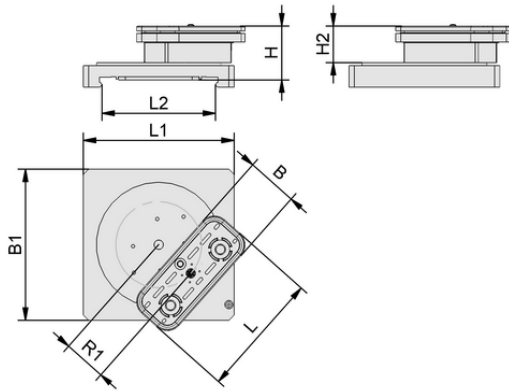
Tasarım verileri VCBL-S4 120x50x50 D-360 TV
