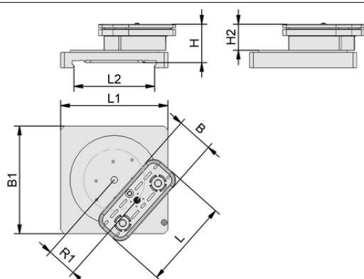
デザインデータ VCBL-S4 120x50x50 D-360 TV
