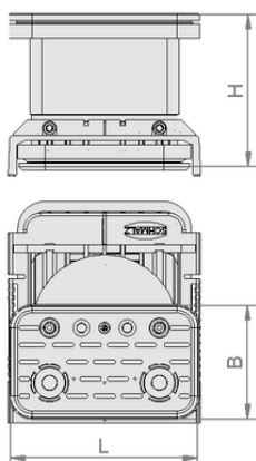
デザインデータ VCBL-K2 125x75x100 D-360
