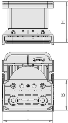
Tasarım verileri VCBL-K2 125x75x100 D-360
