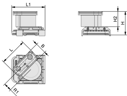
Dati di costruzione VCBL-K2 120x50x100 D-360
