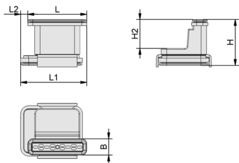
デザインデータ VCBL-K2 130x30x100 L
