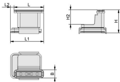
Données de construction VCBL-K2 130x30x100 L
