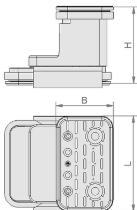
Dati di costruzione VCBL-K2 130x30x100 Q
